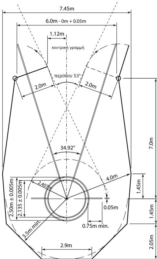
Σχήμα (α) TK37 - Κλωβός για Σφυροβολία και Δισκοβολία με ομόκεντρες βαλβίδες (διαμόρφωση για Σφυροβολία από δεξιόχειρες ρίπτες με διαστάσεις κλωβού για τη δικτύωση)
