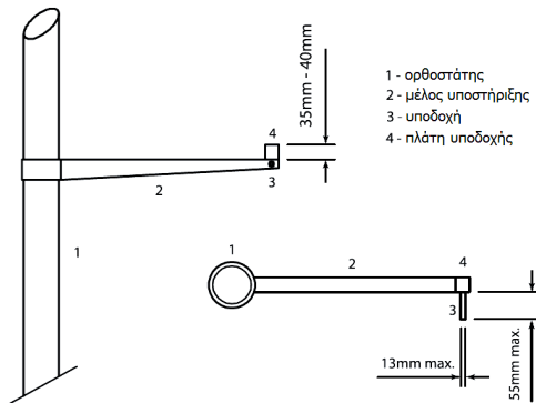
Σχήμα (β) ΤΚ28 (Άρθρο 183): Στηρίγματα πήχη Επί Κοντώ (άποψη από το στρώμα προσγείωσης και κάτωψη)
