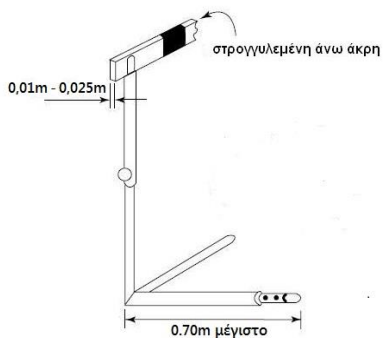
Σχήμα ΤΚ22 (Άρθρο 168) - Παράδειγμα εμποδίου
