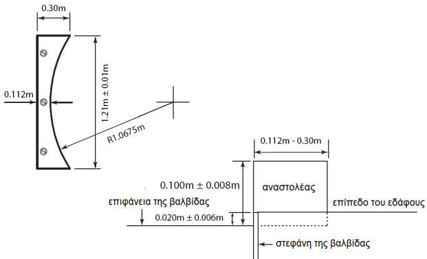
Σχήμα TK33 - Αναστολέας της Βαλβίδας Σφαιροβολίας (κάτοψη και πλάγια όψη)
