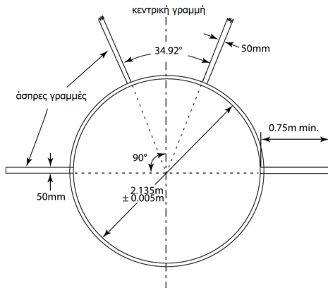
Σχήμα (γ) TK32 - Σχεδίαση της βαλβίδας Σφυροβολίας
