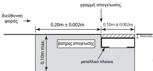
Σχήμα (α1) TK29 - Βατήρας απογείωσης και πλαίσιο ένδειξης από πλαστελίνη
