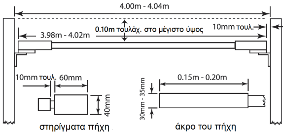
Σχήμα ΤΚ27 (Άρθρο 182) - Στυλοβάτες και πήχης άλματος σε ύψος
