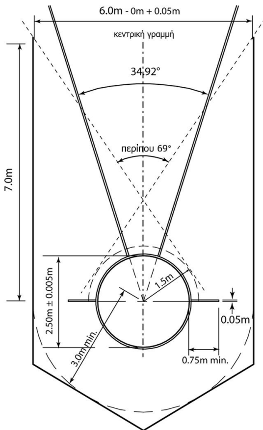
Σχήμα ΤΚ35 - Κλωβός αποκλειστικά για Δισκοβολία (με διαστάσεις κλωβού για τη δικτύωση)
