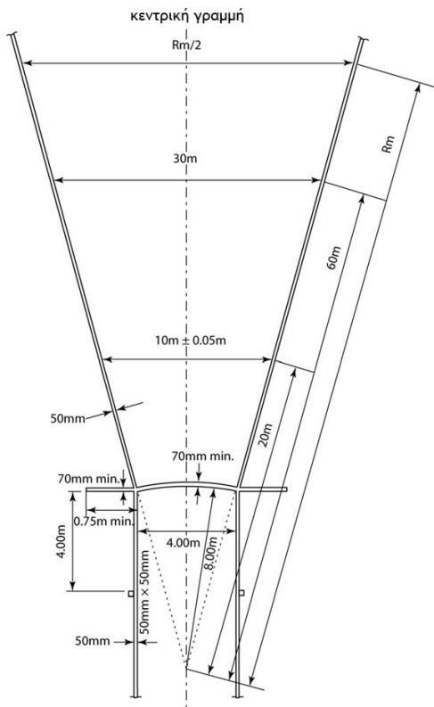
Σχήμα (ε) ΤΚ32: Διάδρομος φοράς και τομέας ρίψης Ακοντισμού (όχι υπό κλίμακα)
