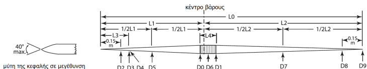
Σχήμα TK38 - Διεθνές Ακόντιο
