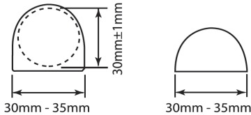
Σχήμα ΤΚ26 (Άρθρο 181) - Εναλλακτικά άκρη πήχη
