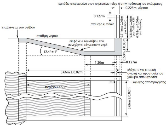
Σχήμα (β) TK23 (Άρθρο 169) - Εμπόδιο λίμνης
