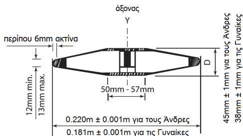
Σχήμα TK34 - Δίσκος
