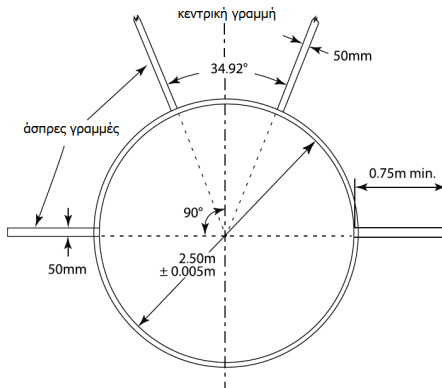
Σχήμα (β) ΤΚ32 - Σχεδίαση της βαλβίδας Δισκοβολίας
