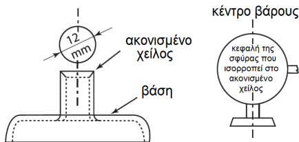
Σχήμα (α) ΤΚ36 - Προτεινόμενη συσκευή για τον έλεγχο του κέντρου βάρους της κεφαλής της σφύρας
