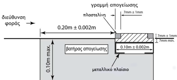
Σχήμα (α2) TK29 - Βατήρας απογείωσης και πλαίσιο ένδειξης από πλαστελίνη
