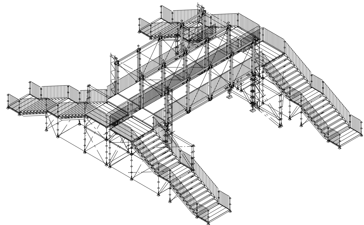
Isometrie
