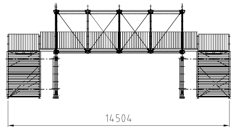
Seitenansicht
