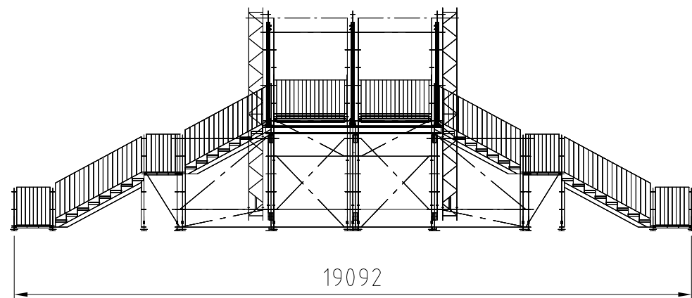
Vorderansicht
