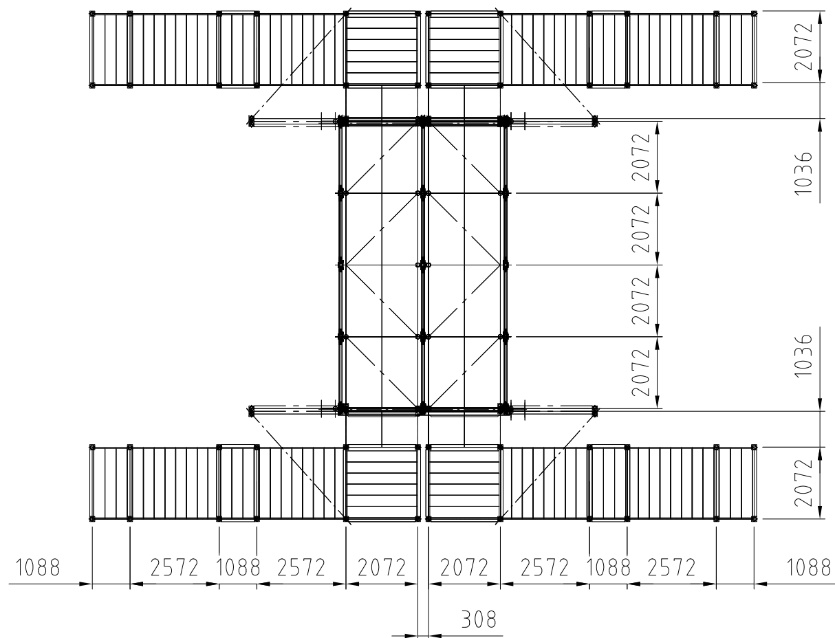
Draufsicht
